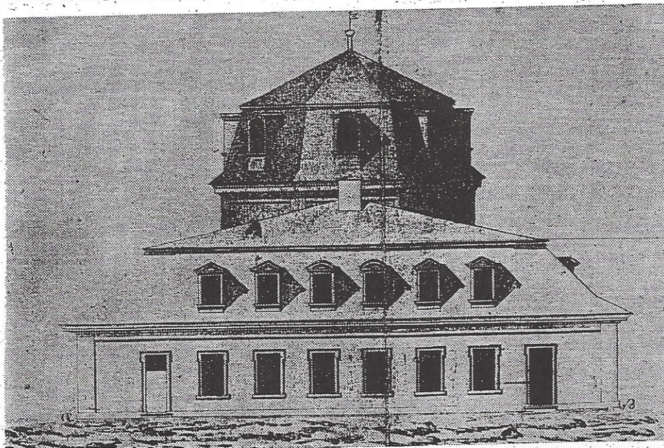
Aufriß des Jagdschlösses (Mittelbau und ein Schloßflügel) nach einem Plan im Besitz des Historischen Vereins für Oberfranken.
